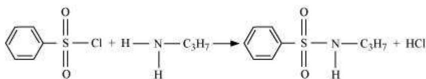
Benzenesulphonyl chloride
